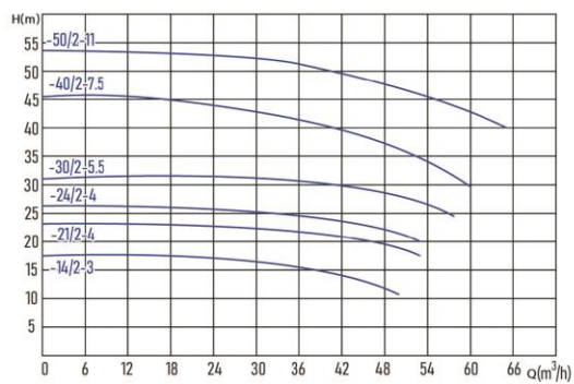
VL2 80
