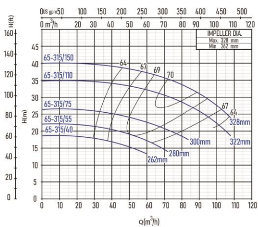
KL 65-315
