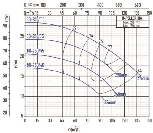
KL 80-250
