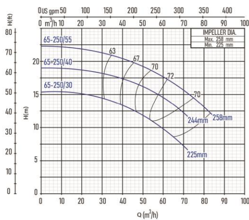
KL 65-250
