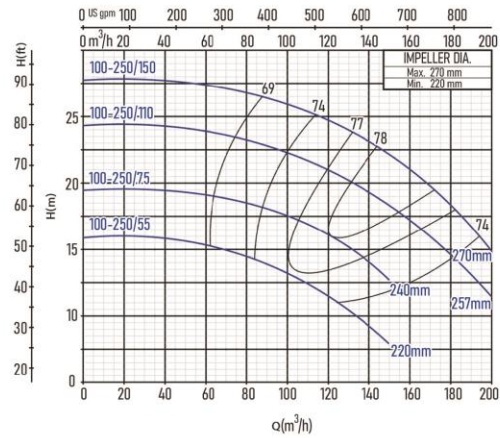
KL4 100-250
