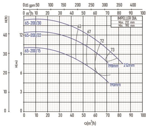
KL 65-200
