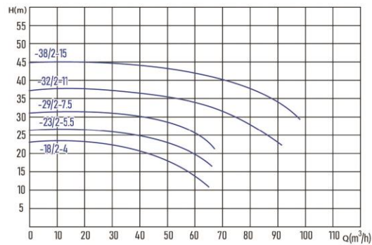
VL2 80
