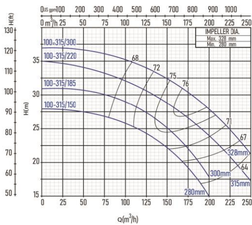
KL4 100-315
