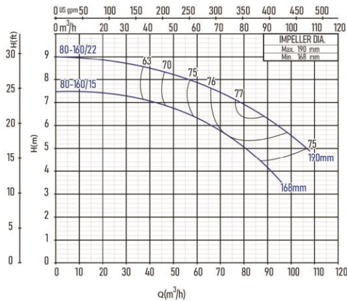
KL 80-160
