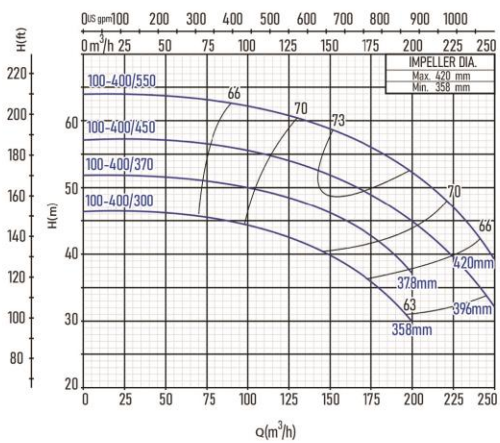
KL4 100-400
