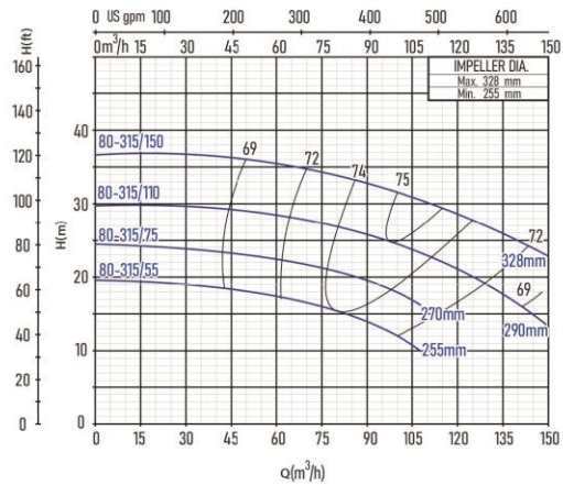
KL 80-315
