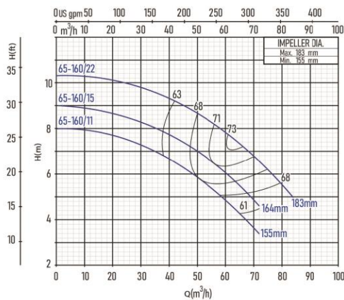
KL 65-160
